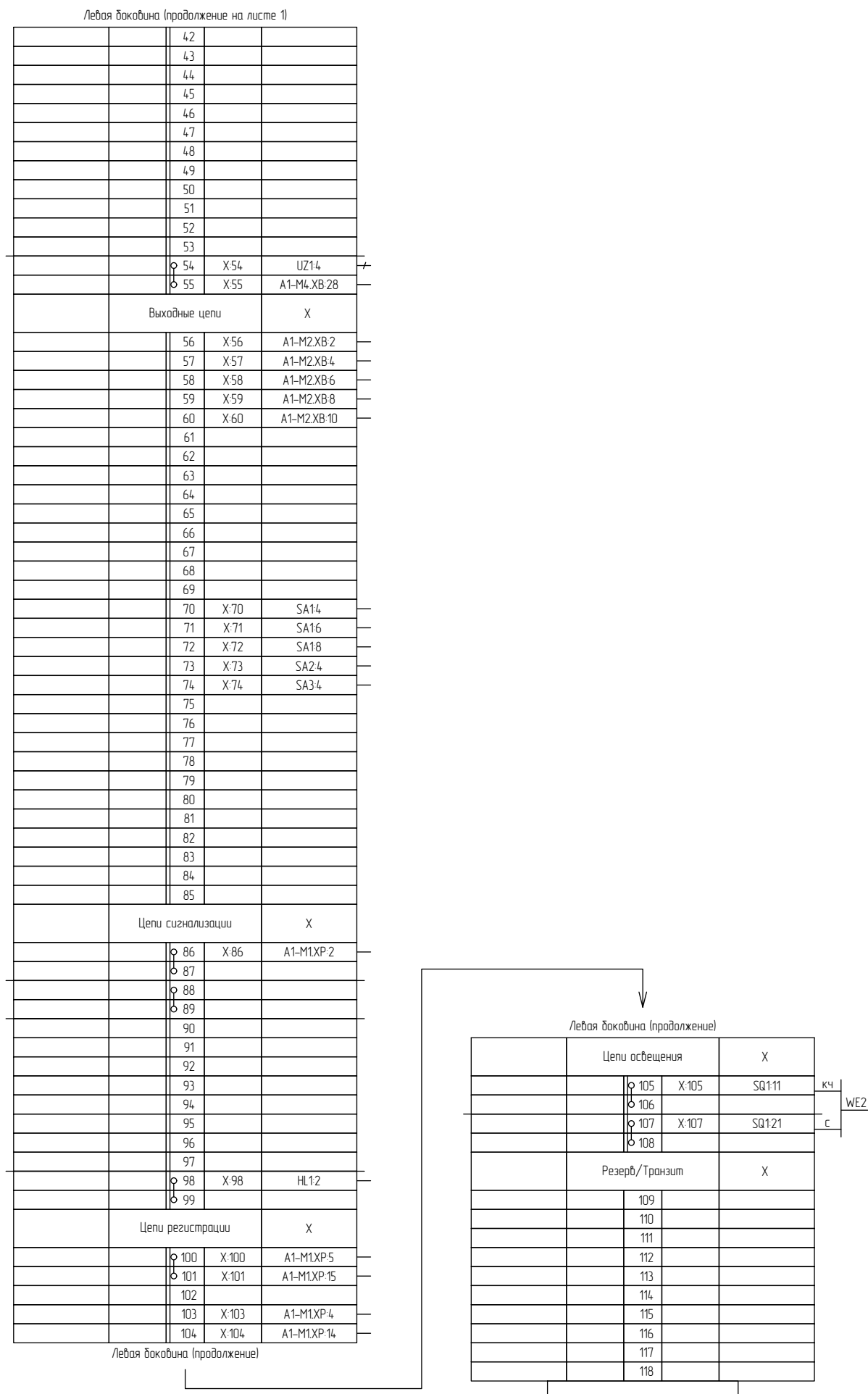
Рисунок Г.2 – Схема электрическая соединений рядов зажимов (часть 2)
